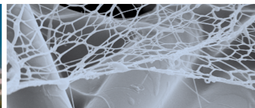
Фильтроматериал Spider-Web при 2500-кратном увеличении. Сетка сверхтонких волокон увеличивает поверхностную пылездерживающую способность и уменьшает количество частиц, проникающих в глубь фильтроматериала.
